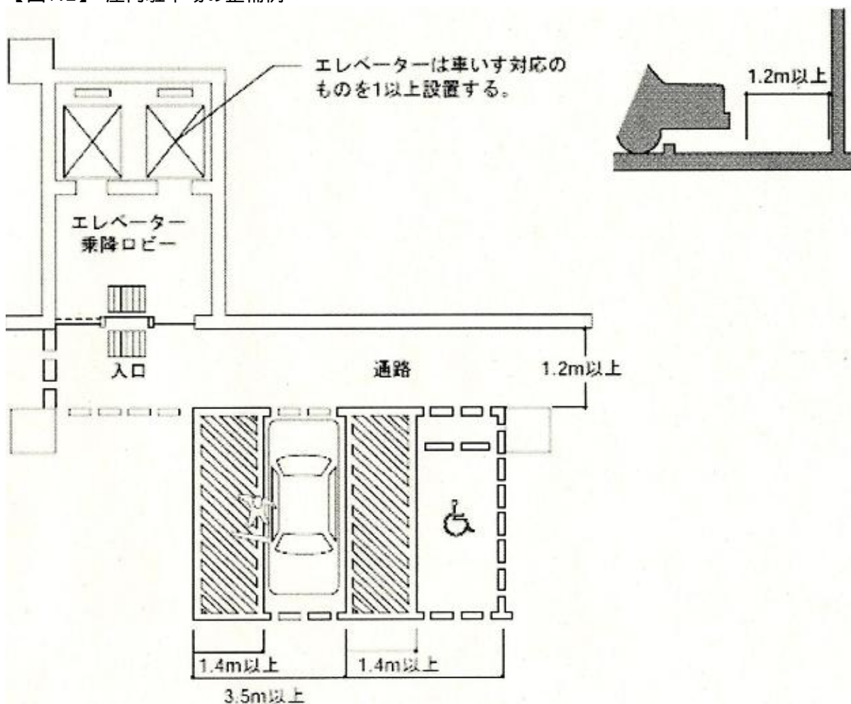
【図1.2】 屋内駐車場の整備例
