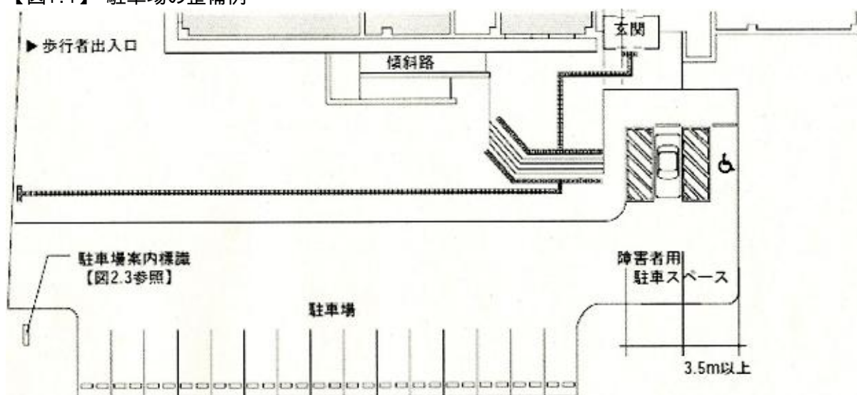
【図1.1】 駐車場の整備例
