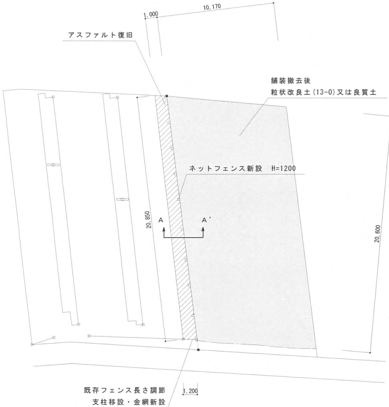
平面図（改修後） 1/200
